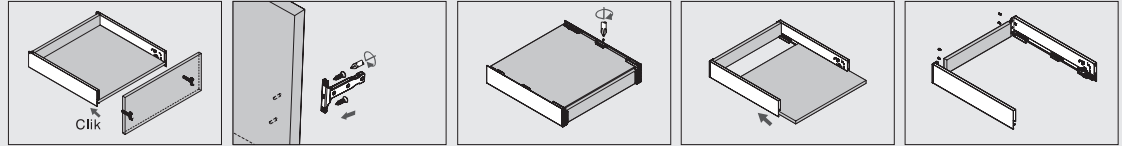
הרכבת חיבור חזית + חזית המגירה
